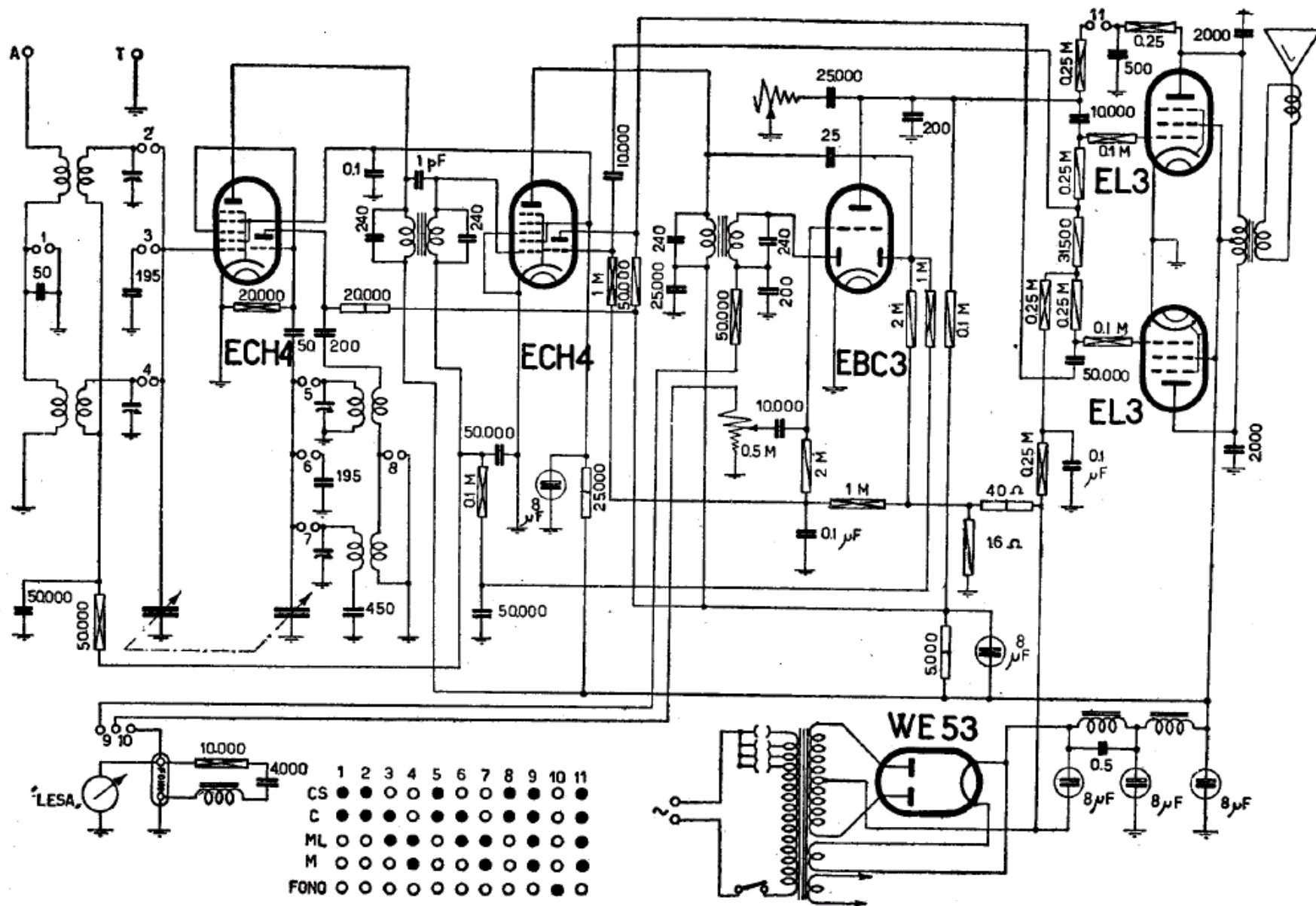
PHONOLA RADIO - Mod. 628 - Quattro gamme, due principali (M e CS) e due spostate (ML e C). Il triodo della seconda ECH4 provvede all'inversione di fase BF. Media frequenza 470 kc/s.
